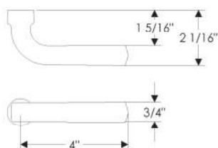
L115 Acanthus Lever
